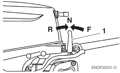
1. Levier inverseur
