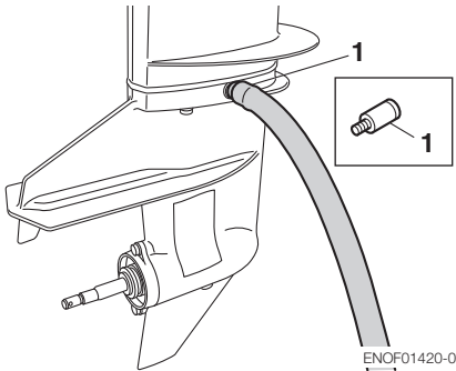
1. Accessoire de rinçage
