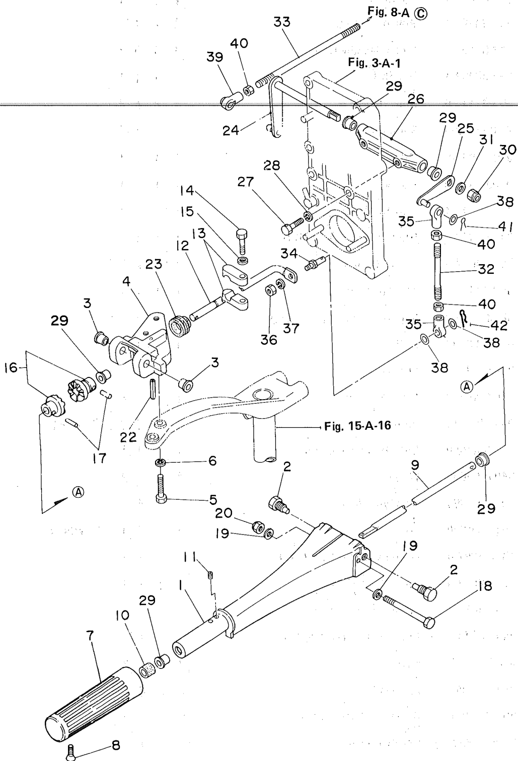
バーハンドル Fig. 9-A BAR HANDLE
