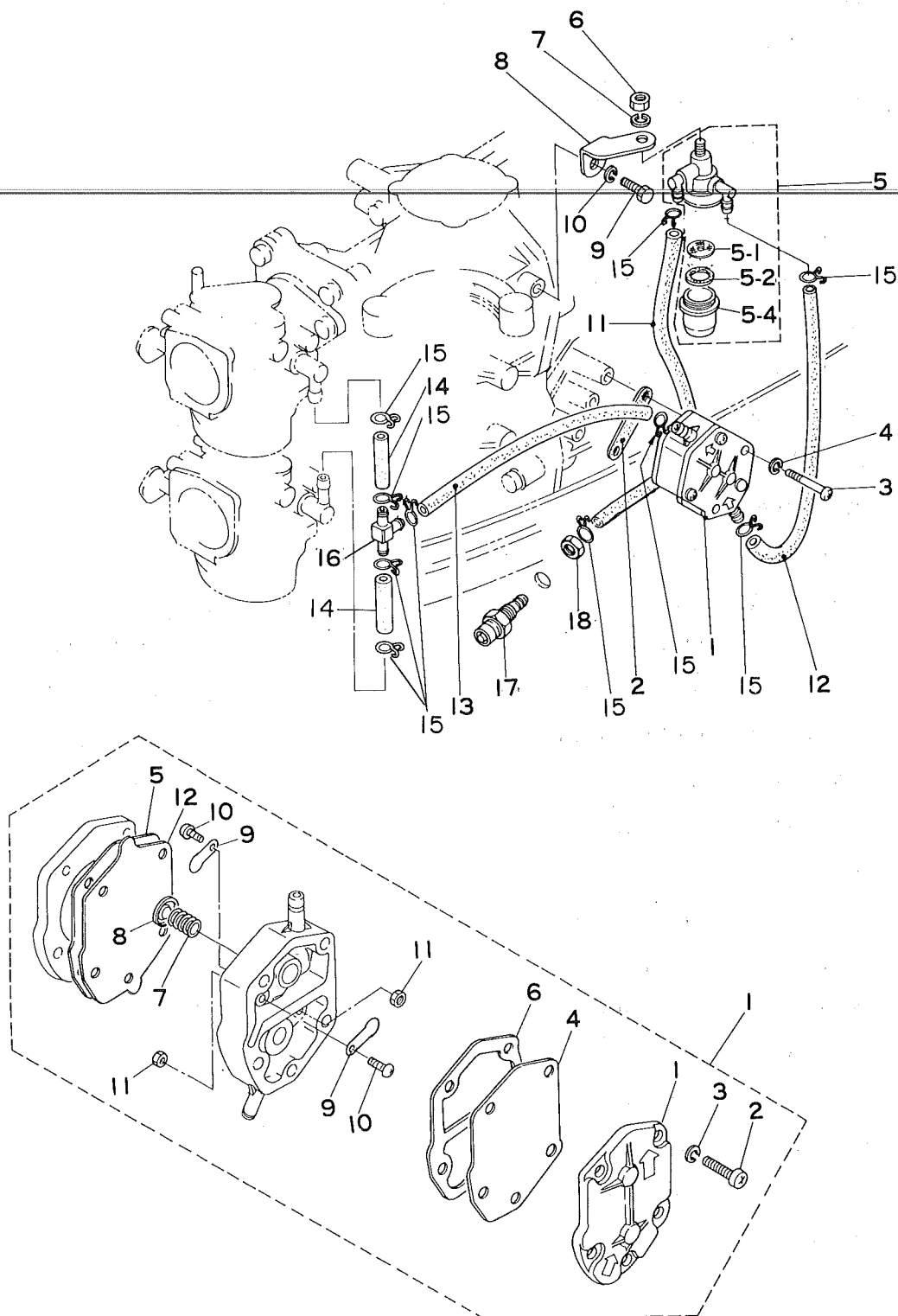
フュエルポンプ Fig. 5-A FUEL PUMP
