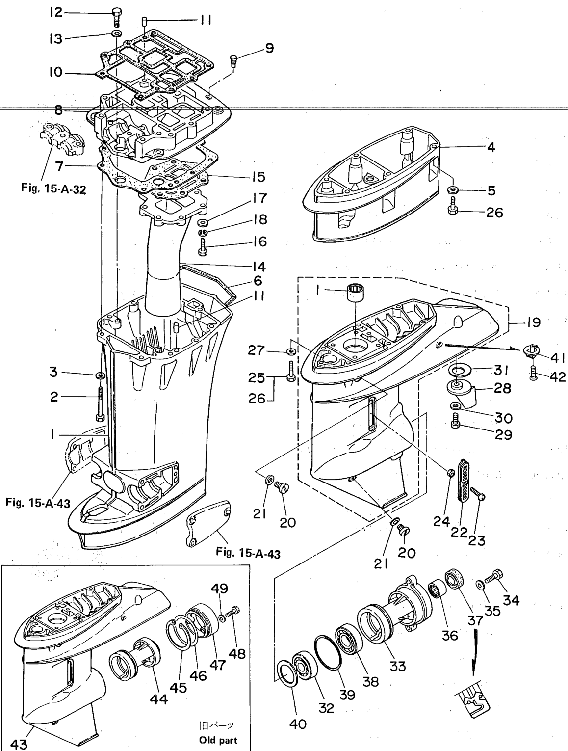
ドライブシャフトハウジング・ギヤケース Fig. 12-A DRIVESHAFT HOUSING・GEAR CASE
