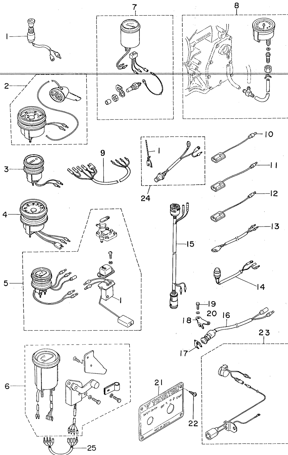
Fig. 20-A OPTIONAL PARTS (III) (Gauges)
