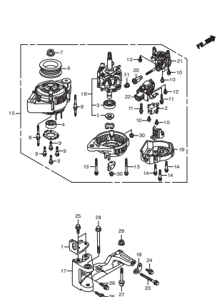
E-19 A.C.GENERATOR
